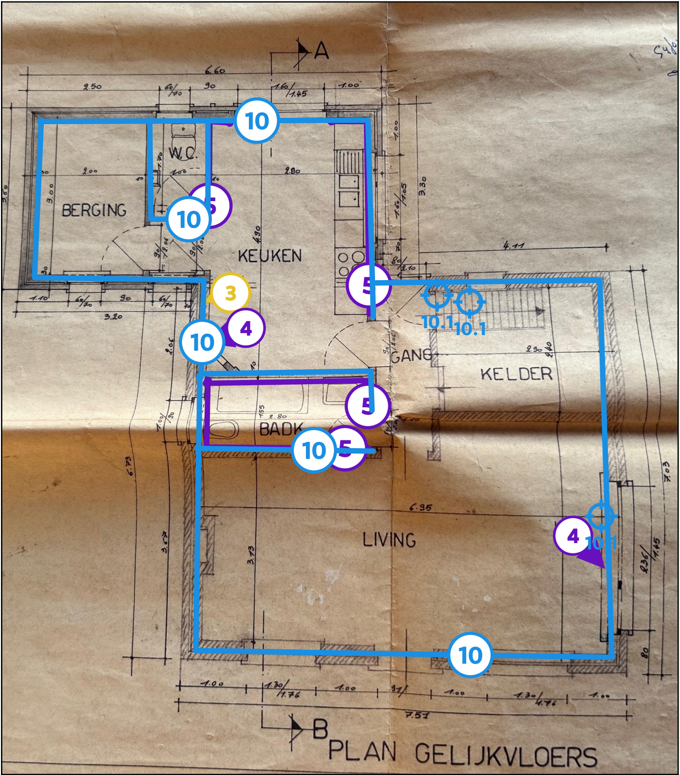
Legende van plan 1.1: Hoofdgebouw: GV
